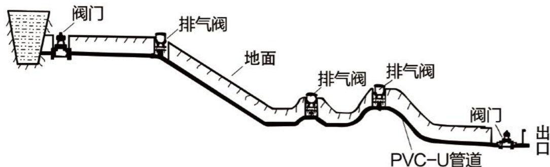
排气阀的安装
