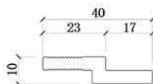
截面图
