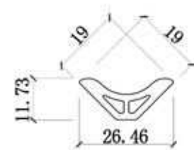
截面图
