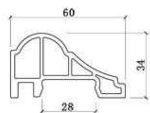
截面图
