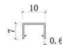
截面图
