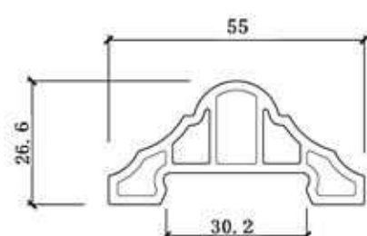
截面图
