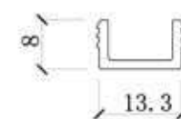
截面图
