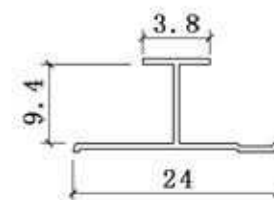
截面图
