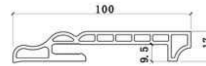
截面图
