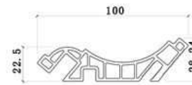
截面图
