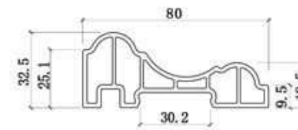
截面图
