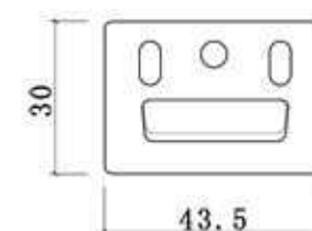
截面图
